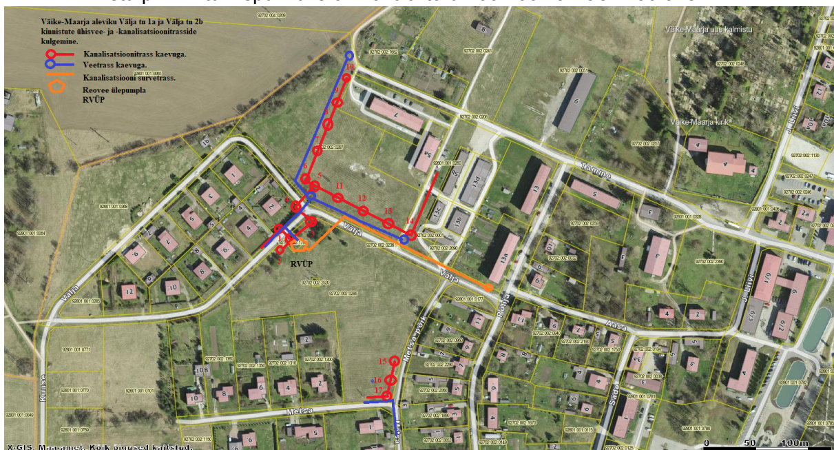
Skeem 3. Pandivere Vesi OÜ poolt koostatud skeem olemasolevate vee ja kanalisatsiooni trasside ning rajatiste põhimõttelise paiknemise kohta.
